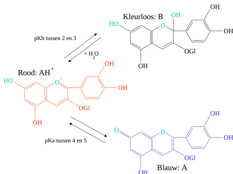
Figuur 6: Drie vormen van anthocyanine \text{AH}^+ , A en B .
