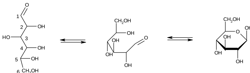
Figuur 2: de reactie van de lineaire vorm van glucose tot \beta -glucopyranose.
