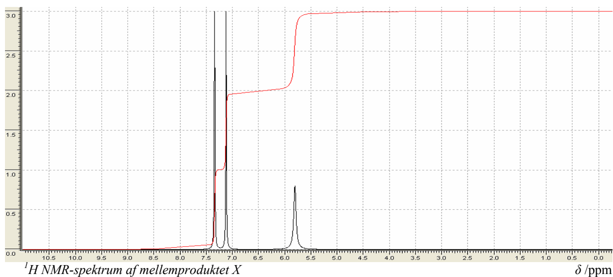
^1\text{H} NMR-spektrum af 1,2,4,5-tetrachlorbenzen
